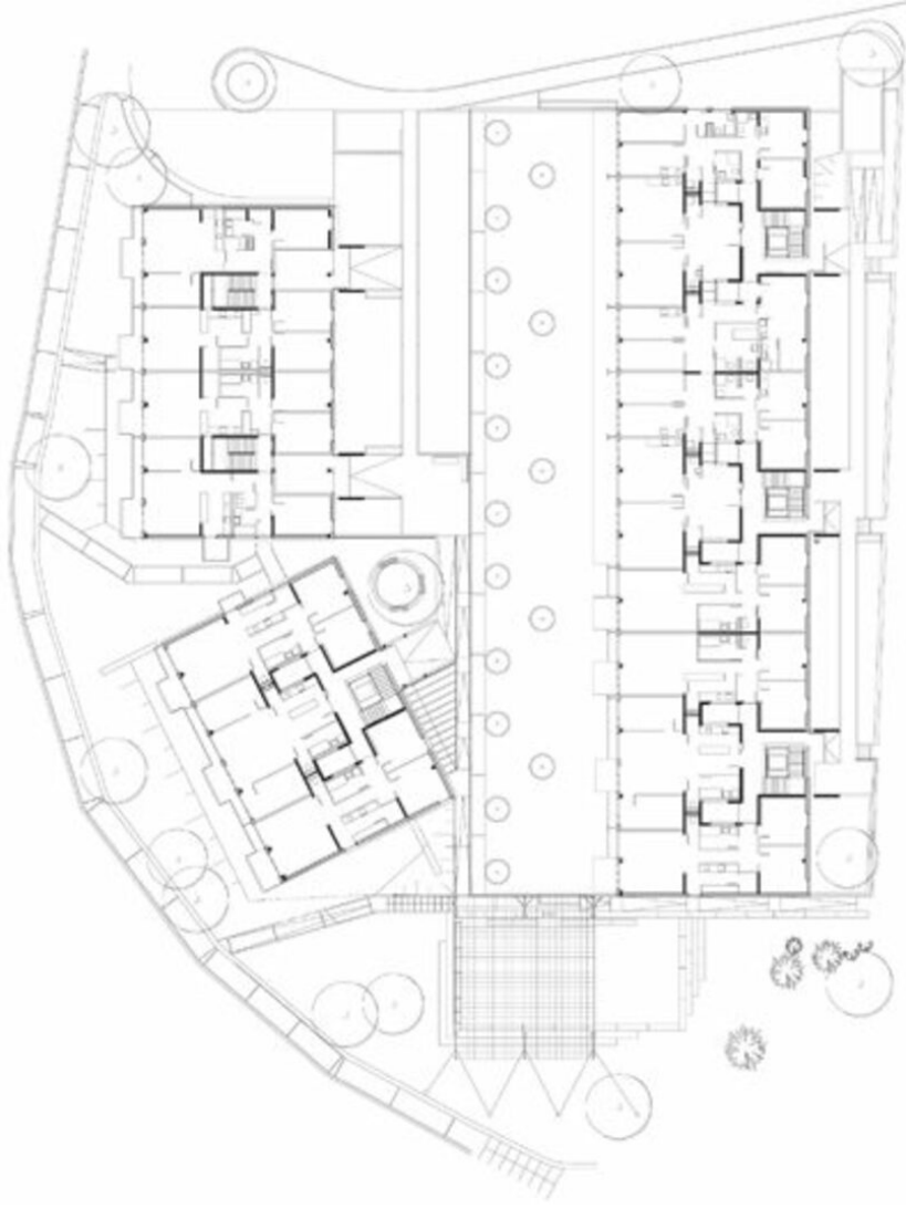
Grundriss EG
