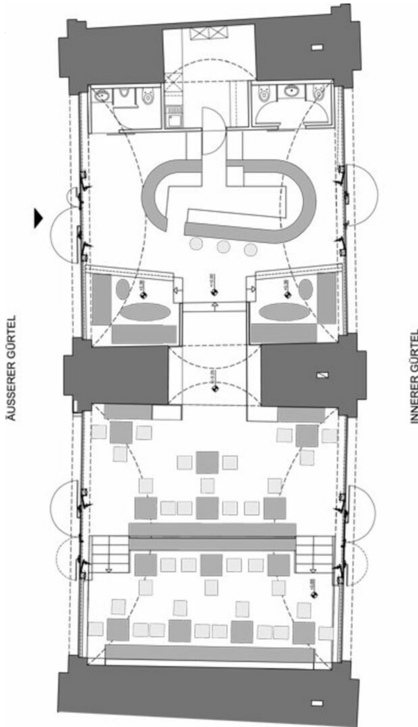
Grundriss
