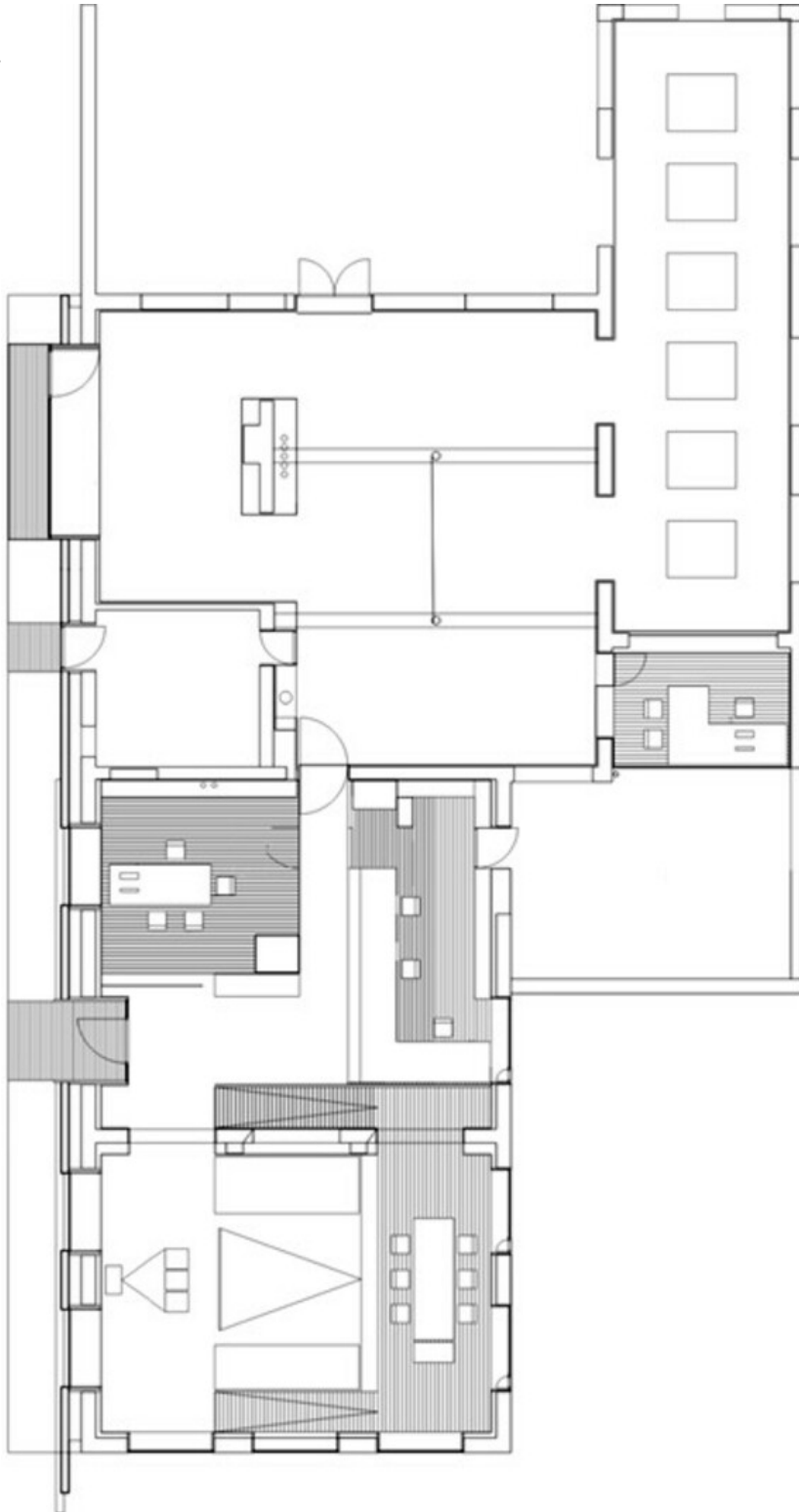
Grundriss EG
