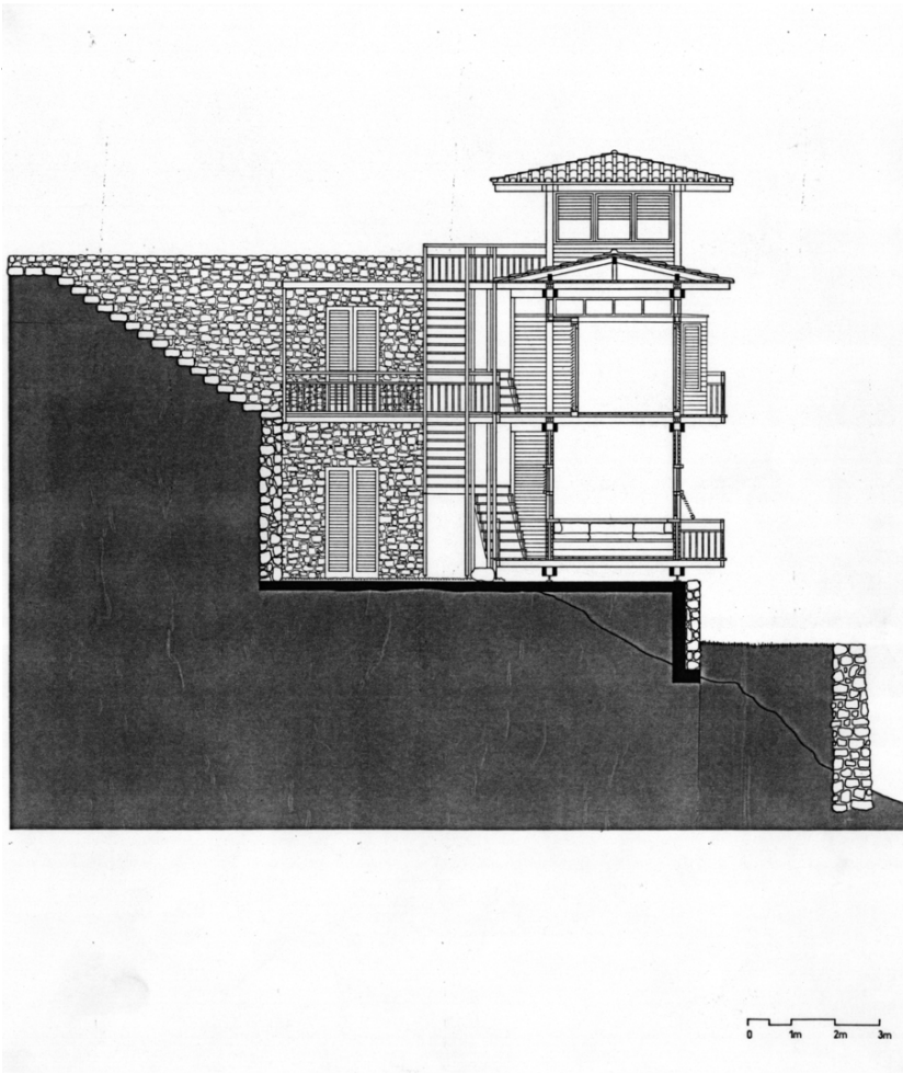
Querschnitt
