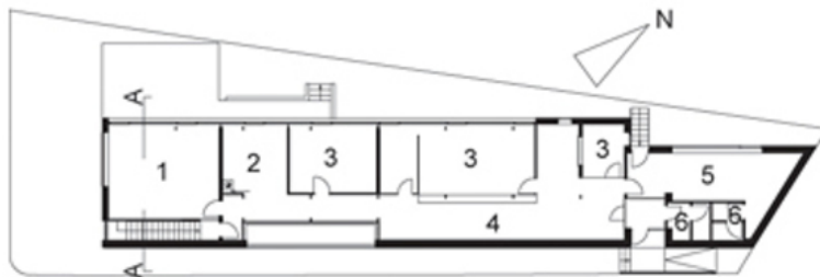
GRUNDRISS ERDGESCHOSS
