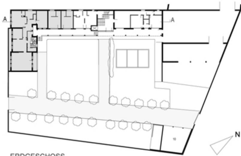
ERDGESCHOSS
