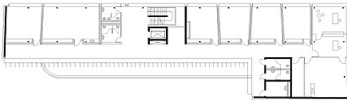
1. OBERGESCHOSS
