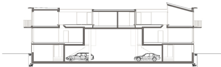
QUERSCHNITT
