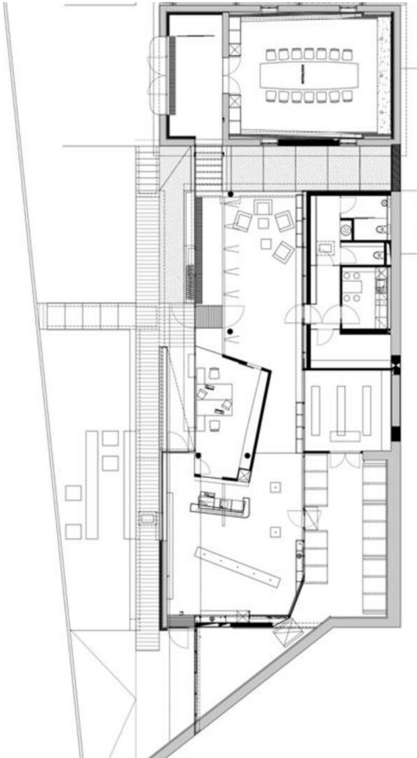
Grundriss EG
