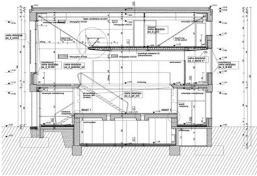
Schnitt
