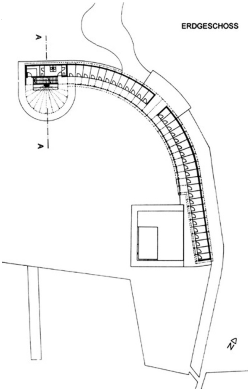
Grundriss EG
