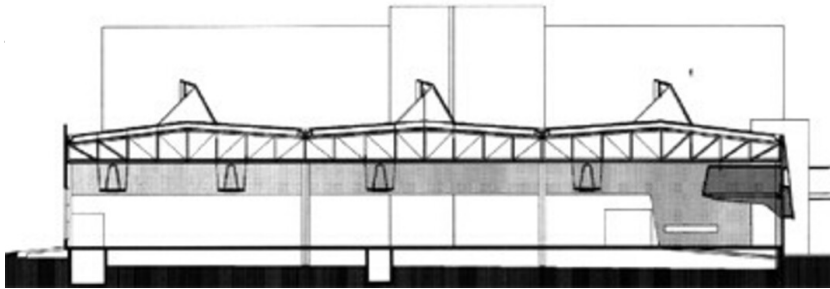
Schnitt Produktionstrakt
