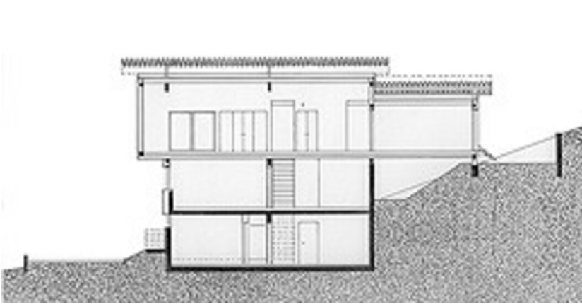
Längsschnitt
