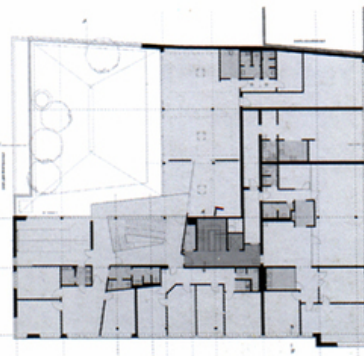
Pôdorys 3. NP
