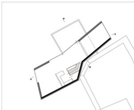
GRUNDRISS OBERGESCHOSS
