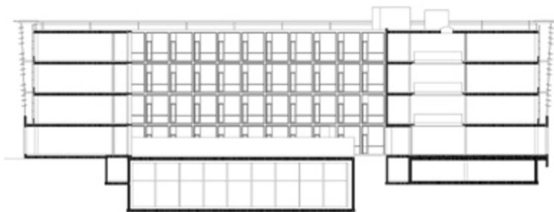
SNITT 1:200
