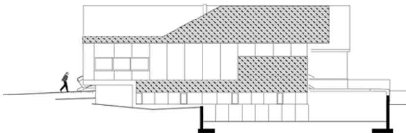
0 1 2 5 ANSICHT SÜD
