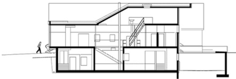
0 1 2 5 LÄNGSSCHNITT
