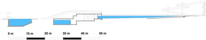
Schnitt
