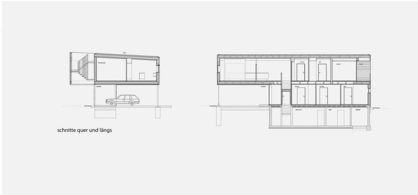
Schnitte
