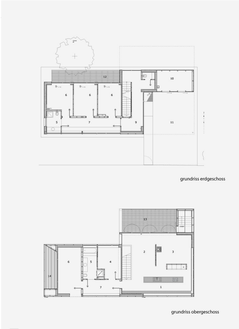
Grundriss
