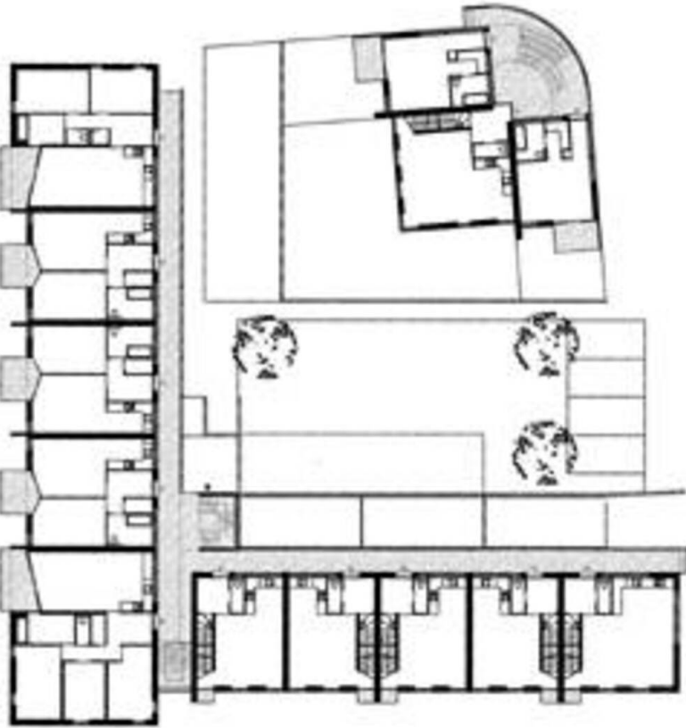
Grundriss EG
