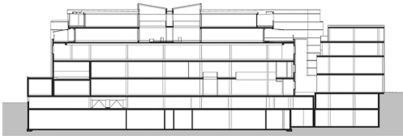
Lageplan, Schnitt
