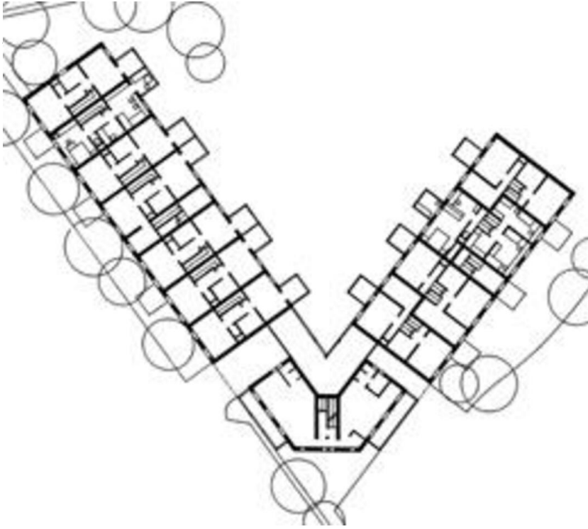
Grundriss EG
