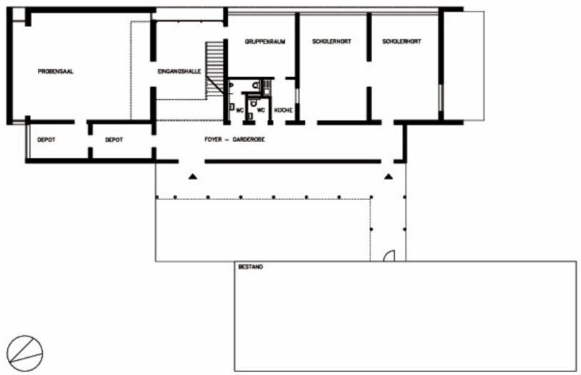
Grundriss EG
