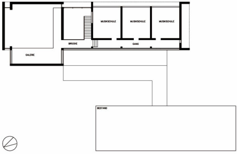
Grundriss OG
