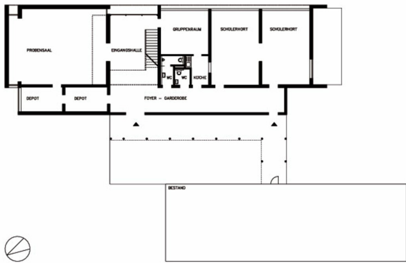
Grundriss EG
