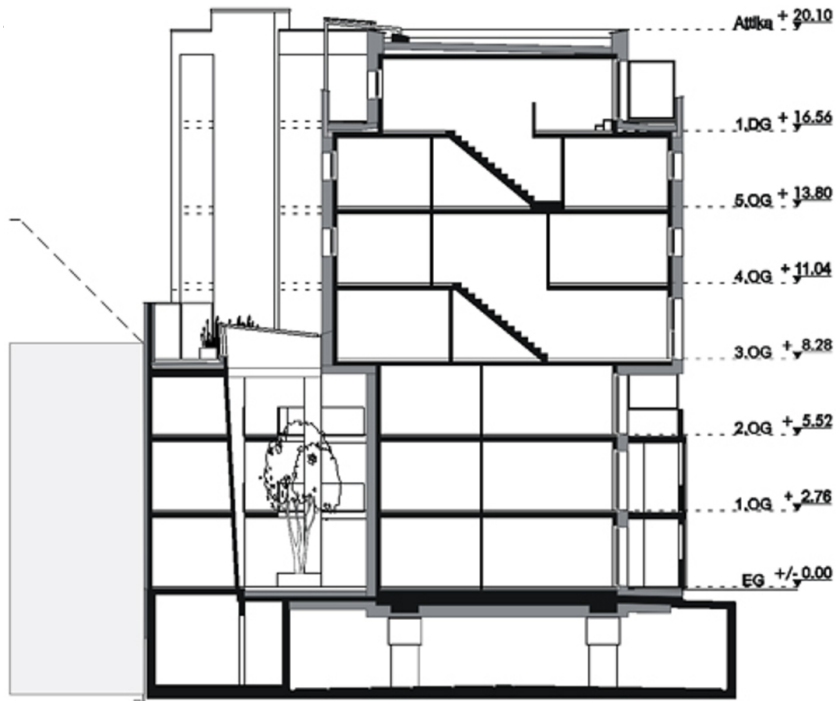
Schnitt
