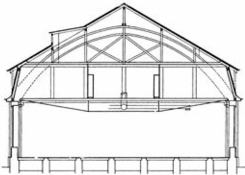
Schnitt
