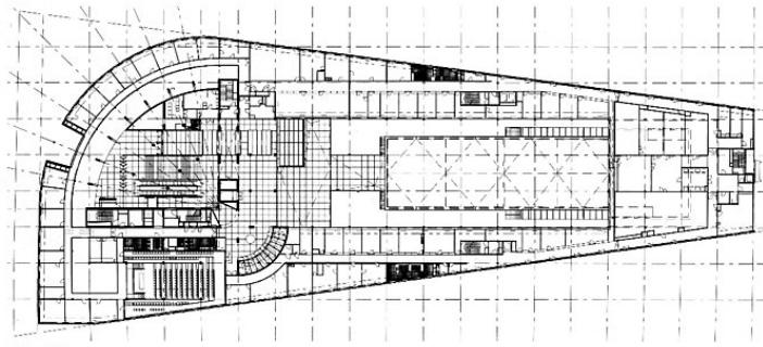
Pôdorys 2. NP
