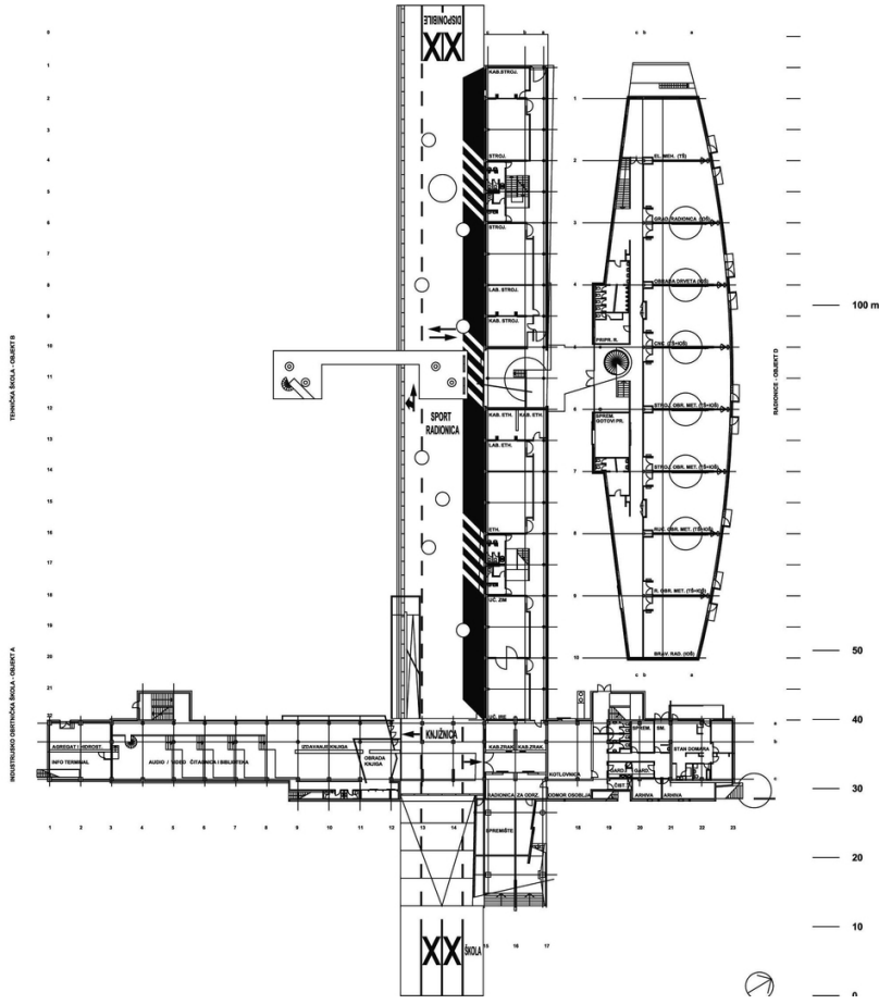
Grundriss EG
