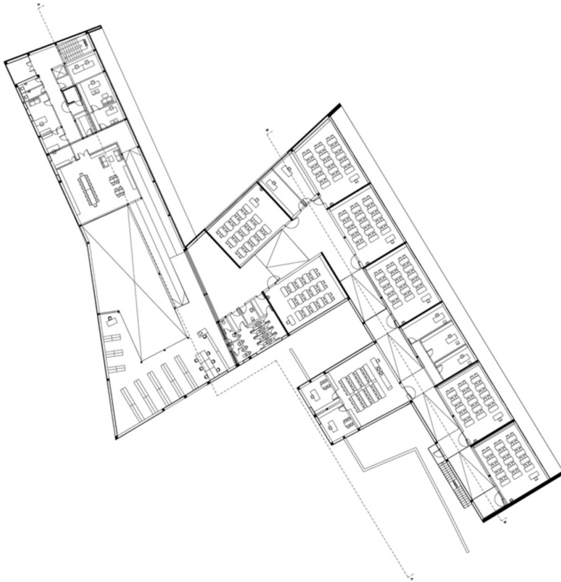
Grundriss EG
