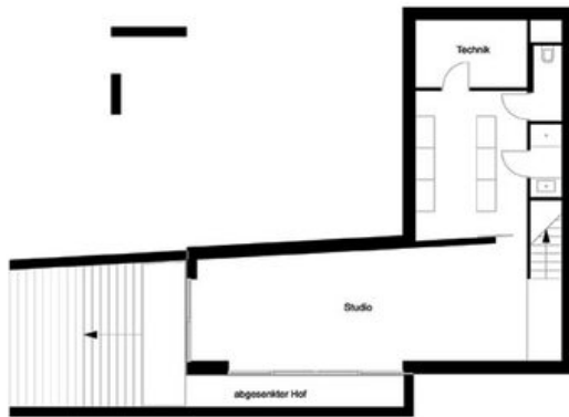
Grundriss Untergeschoss
