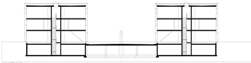
SCHNITT QUER
