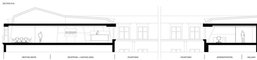
Schnitt B-B
