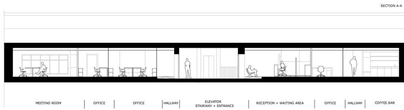
Schnitt A-A
