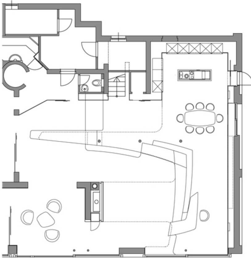
Grundriss EG
