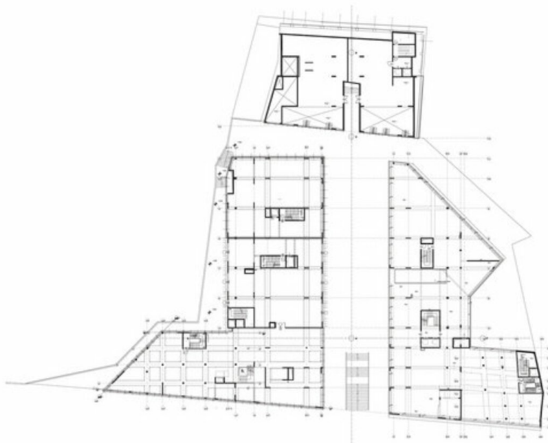
Grundriss OG1
