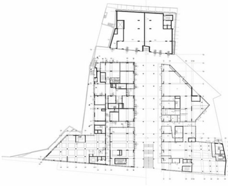
Grundriss EG
