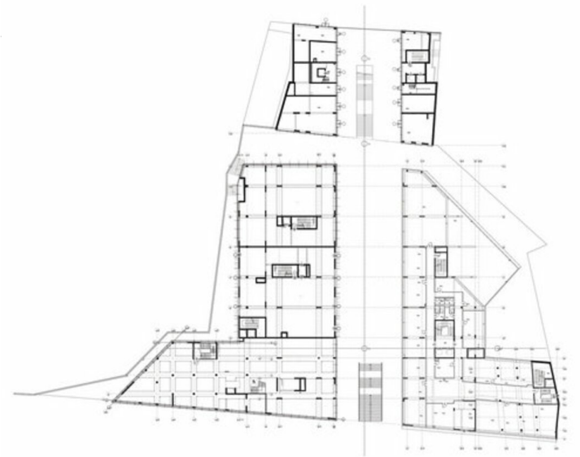
Grundriss OG2
