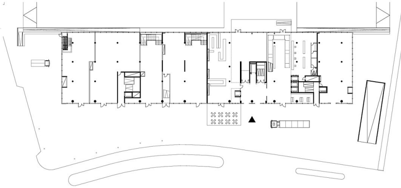
ERDGESCHOSS M 1:500
