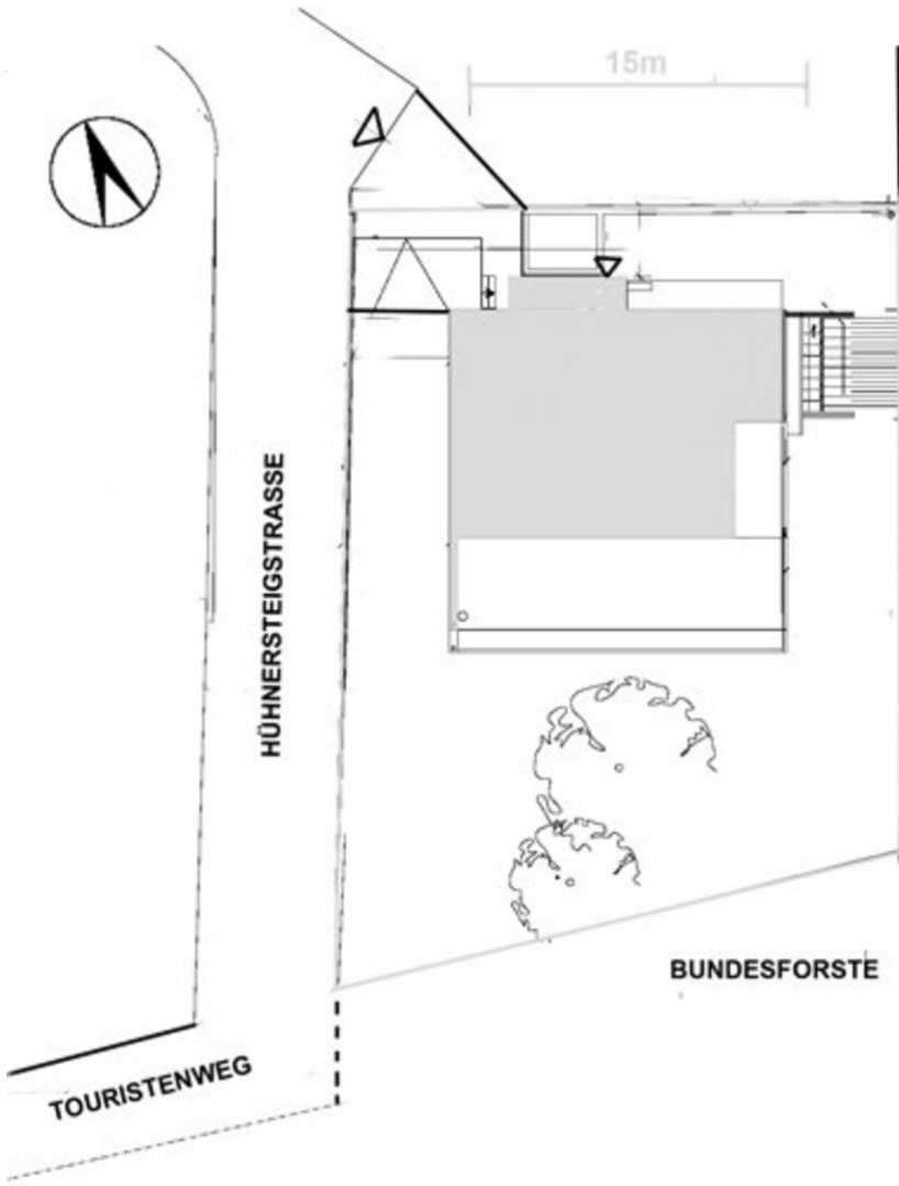
Einfamilienhaus KS
