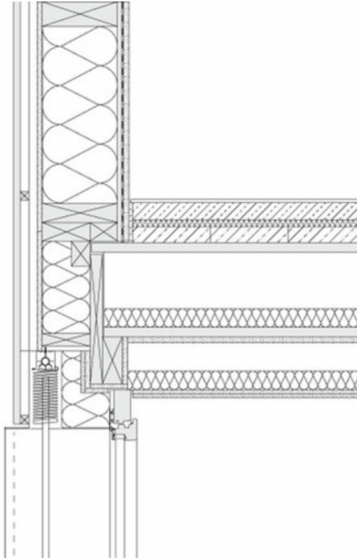
Fassadenschnitt
