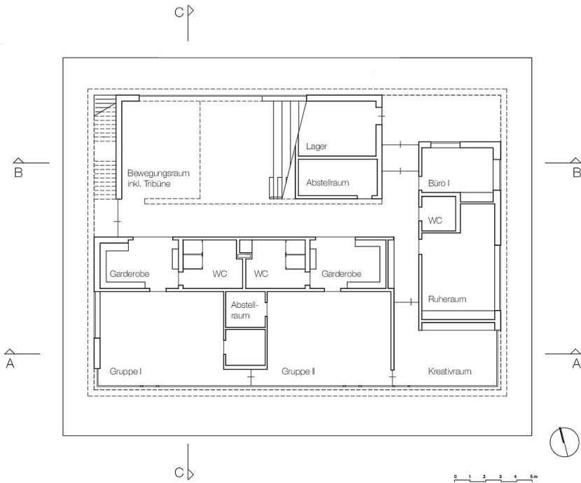
Grundriss Erdgeschoss
