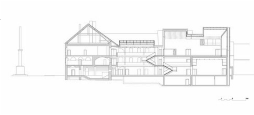
Längsschnitt
