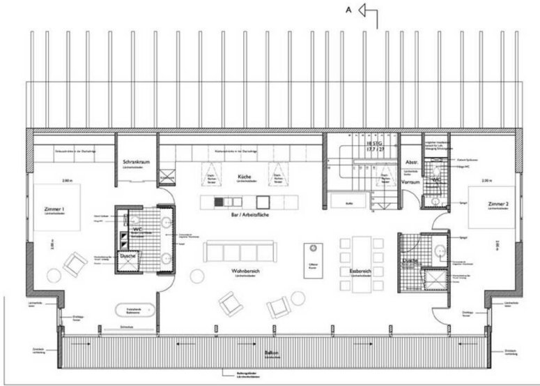
Grundriss Dachgeschoss
