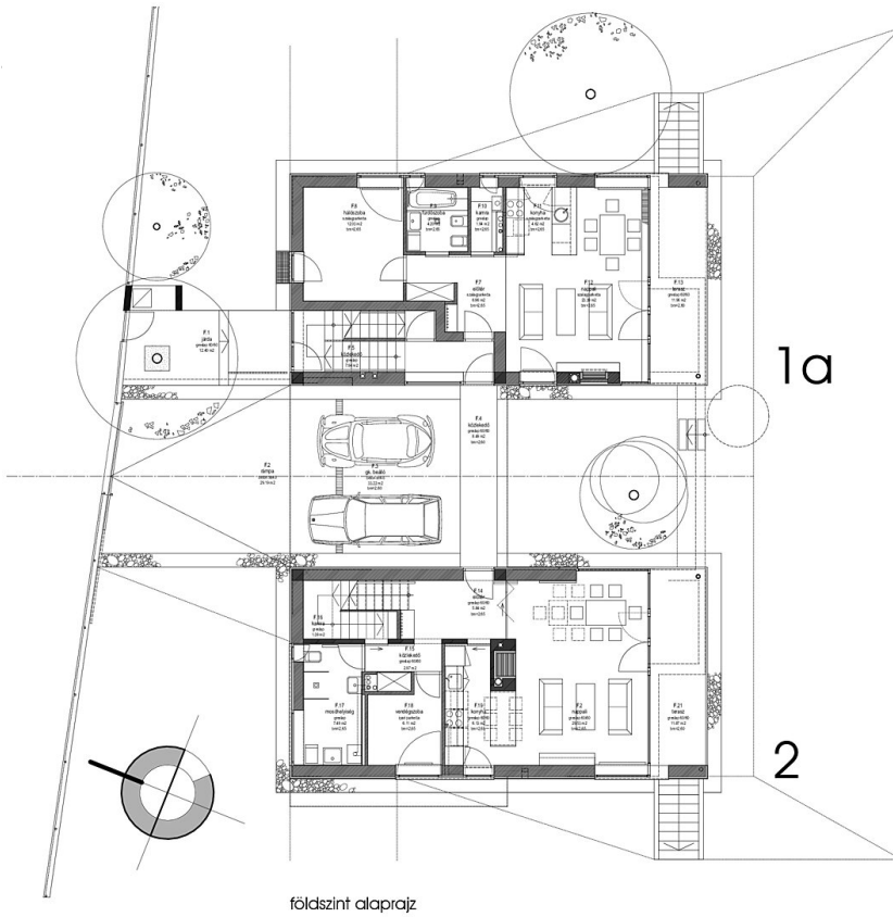
földszint alaprajz
