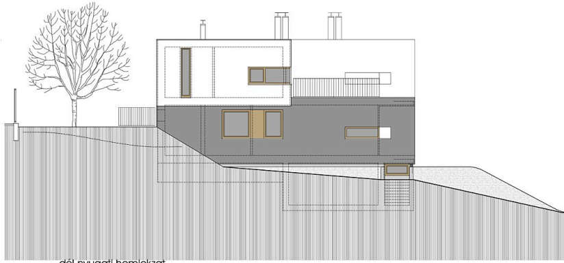
dél-nyugati homlokzat
