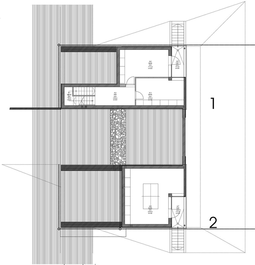
alagsor alaprajz
