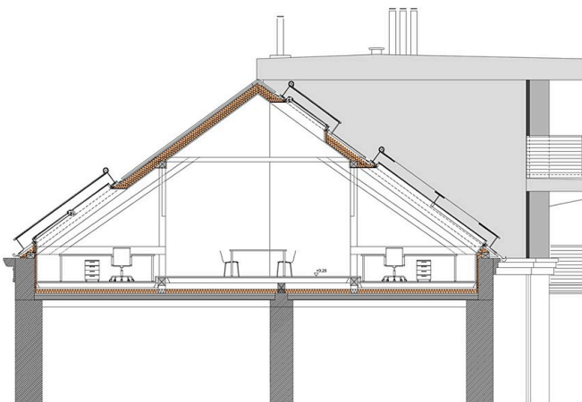
Muchargasse 30 Schnitt 2
