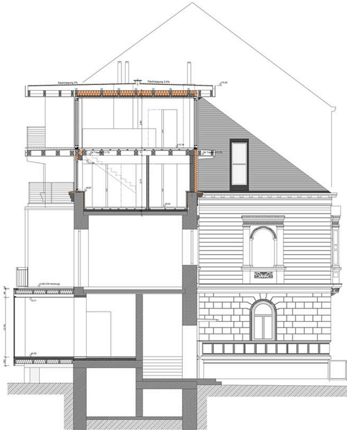
Muchargasse 30 Schnitt 1
