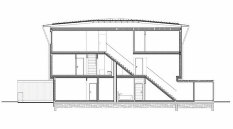
Schnitt
