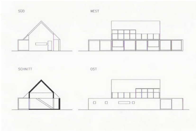
Ansichten, Schnitt
