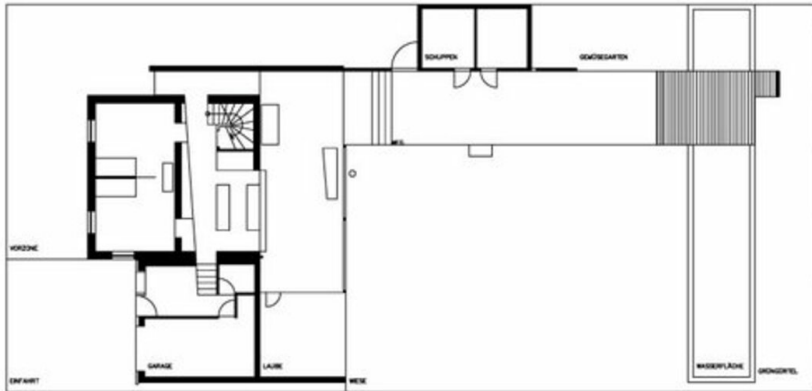
Grundriss
