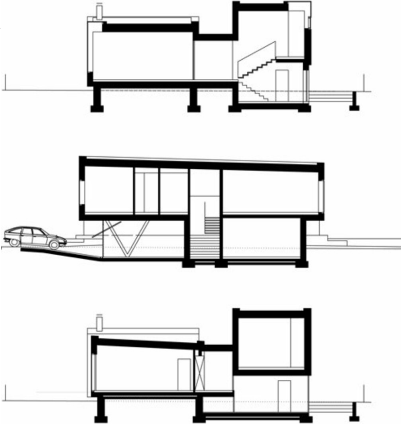
Schnitte
