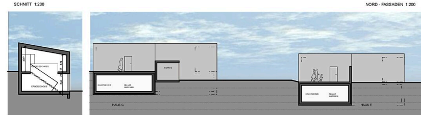
Fassaden Ost Nord
