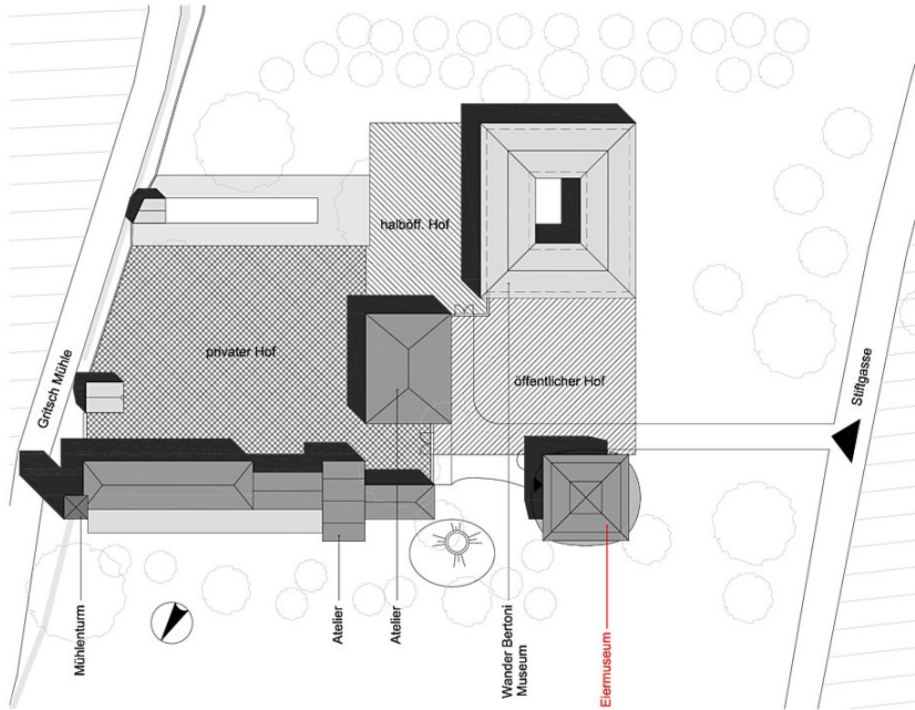
Lageplan & Ansicht
