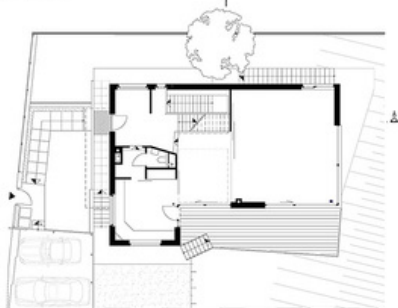
Erdgeschoss
