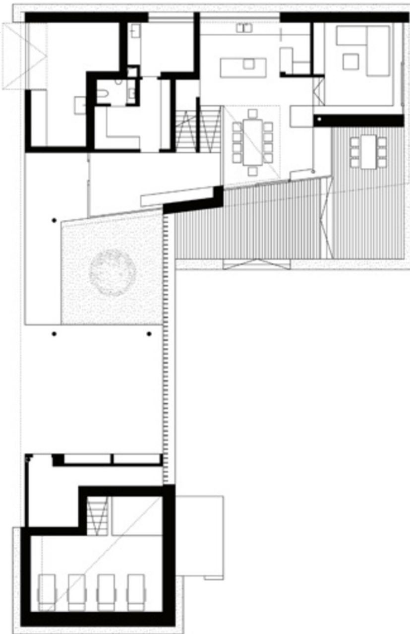
Grundriss EG
