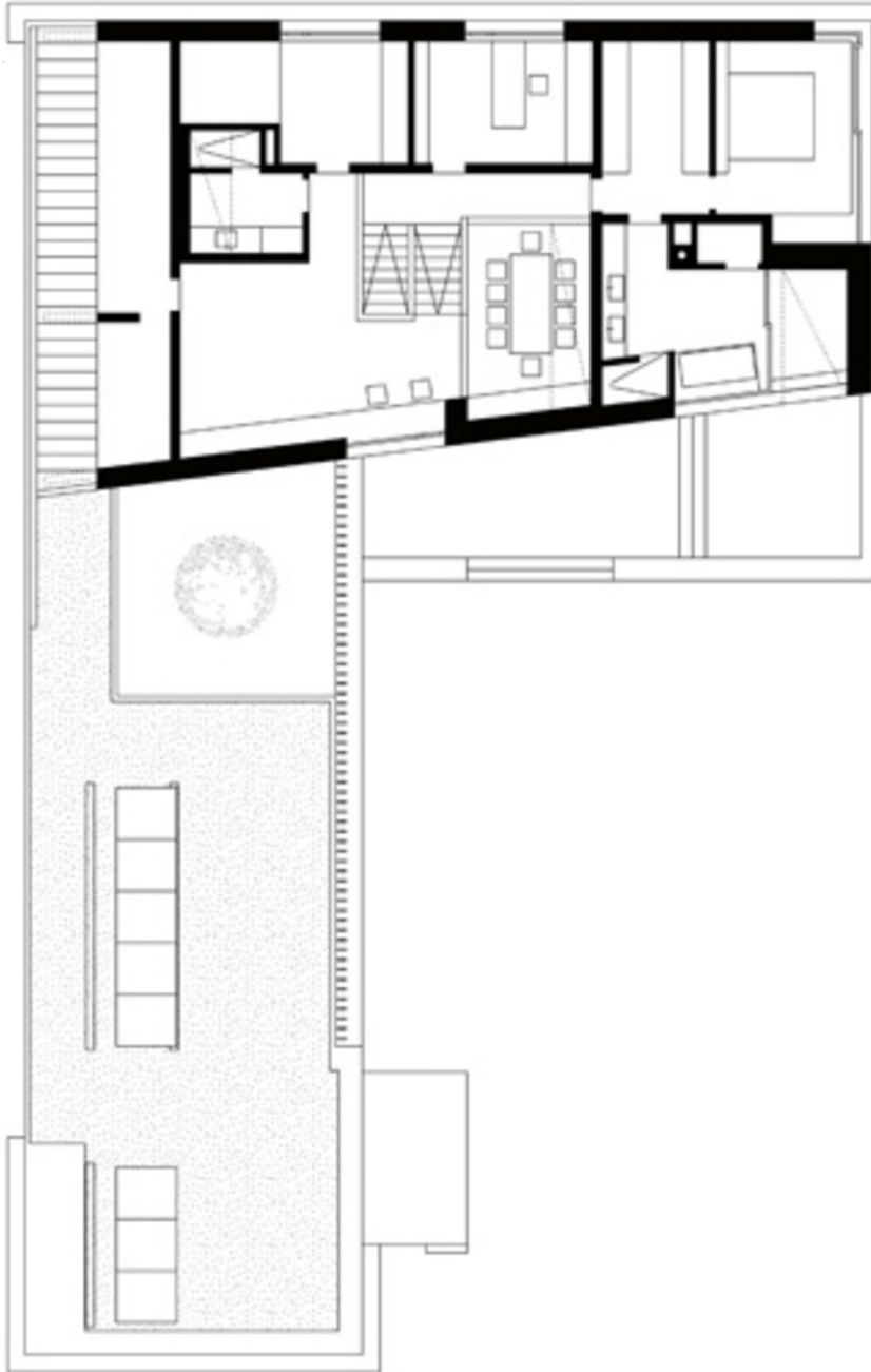
Grundriss OG
