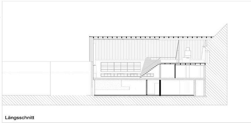
Längsschnitt
